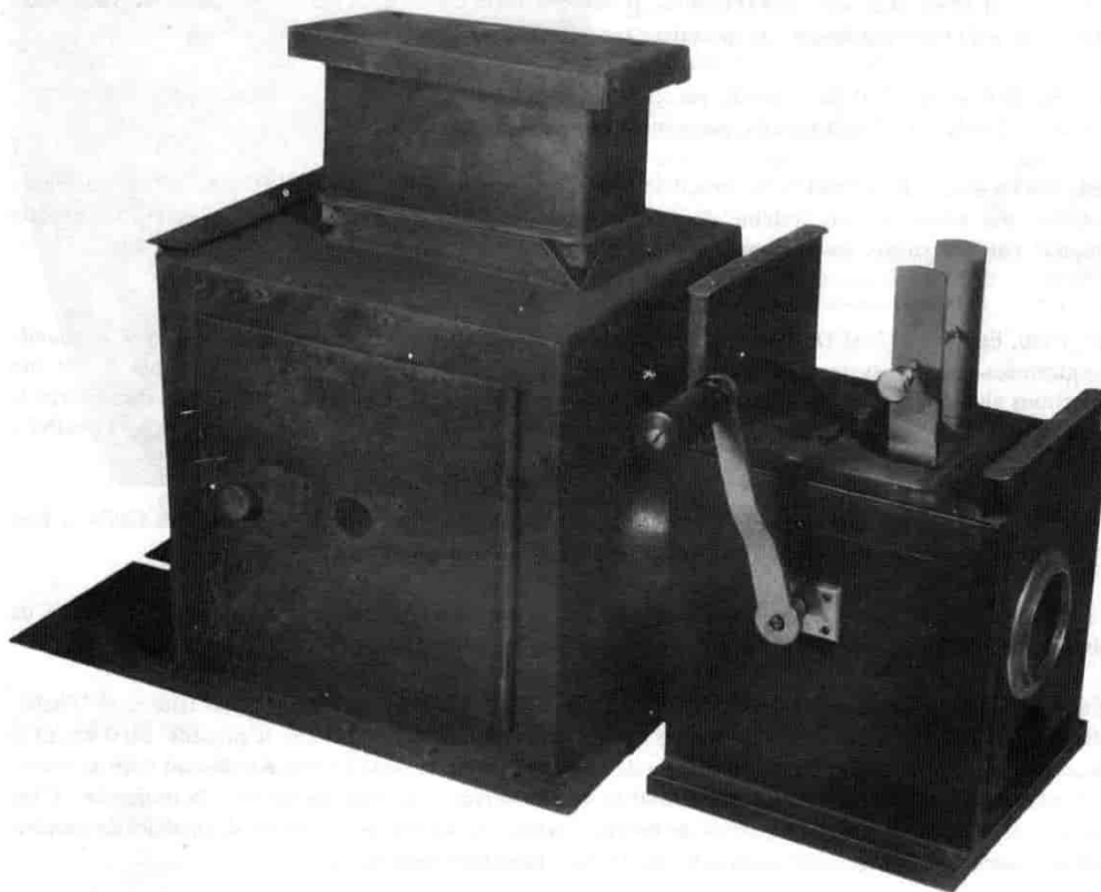
Modèle de LAPIPOSCOPE pour projection avec lanterne d'éclairage à arc, film 35 mm
