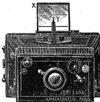
Décentrement vers le bas
