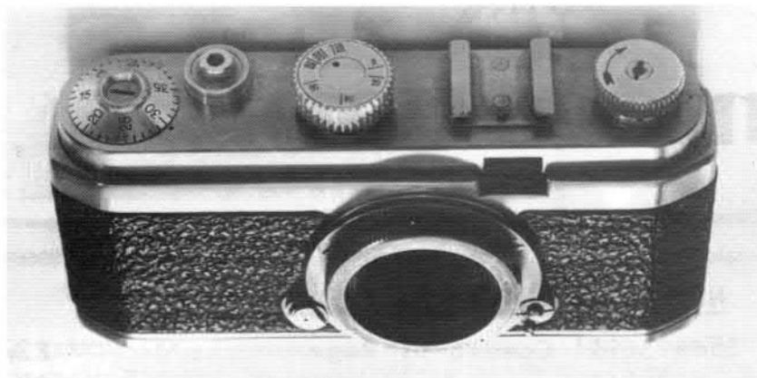
Vue montrant le compteur typiquement FOCA et le bouton d'armement gradué B-20-30-50-100-200-600-
