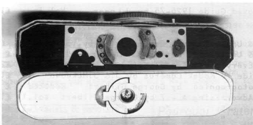
Système de fixation du dos identique à celui du modèle définitif. Noter à gauche l'astucieux principe de blocage des vis de réglage des rideaux. En fait, le procédé retenu ( clip s'engageant dans les fentes des vis ) a l'avantage de permettre un réglage demi-tour par demi-tour.
