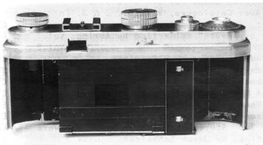
PROTOTYPE DOS RETIRE. Remarquer le cache, fait de 4 lames métalliques croisées, collé sur la fenêtre 24X36, l'oculaire rectangulaire encastré; et le mécanisme tenu seulement par 4 vis ( 6 par la suite ).
