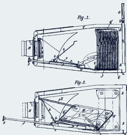
1896 - Plan du brevet n° 253307 Société C. Mercier & A. Millot
