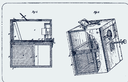
1891 - Plan du brevet n° 217129 Commercialisé sous le nom « Tri-Octo » Société C. Mercier & A. Dumont
