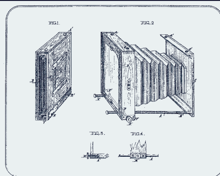
1890 - Plan du brevet n° 210819 Société C. Mercier & A. Dumont Commercialisé sous le nom « Photo-Vélo »
