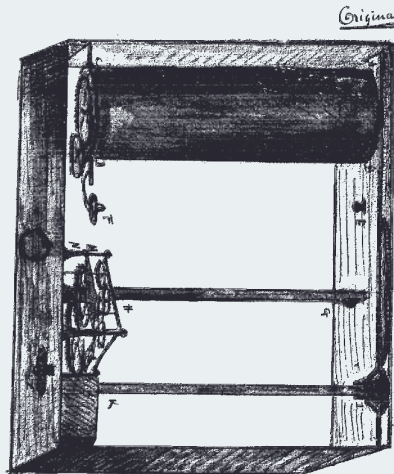
1897 - Magasin pelliculaire à avancement automatique de la pellicule. Brevet n° 270738 du 29 septembre 1897 Auguste Dumont à Tourcoing.
